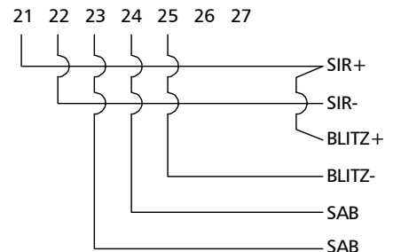
Abb. 24 : Beispiel mit AS 14
