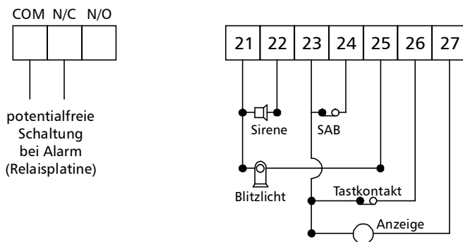
Abb. 21 : Anschlussübersicht
