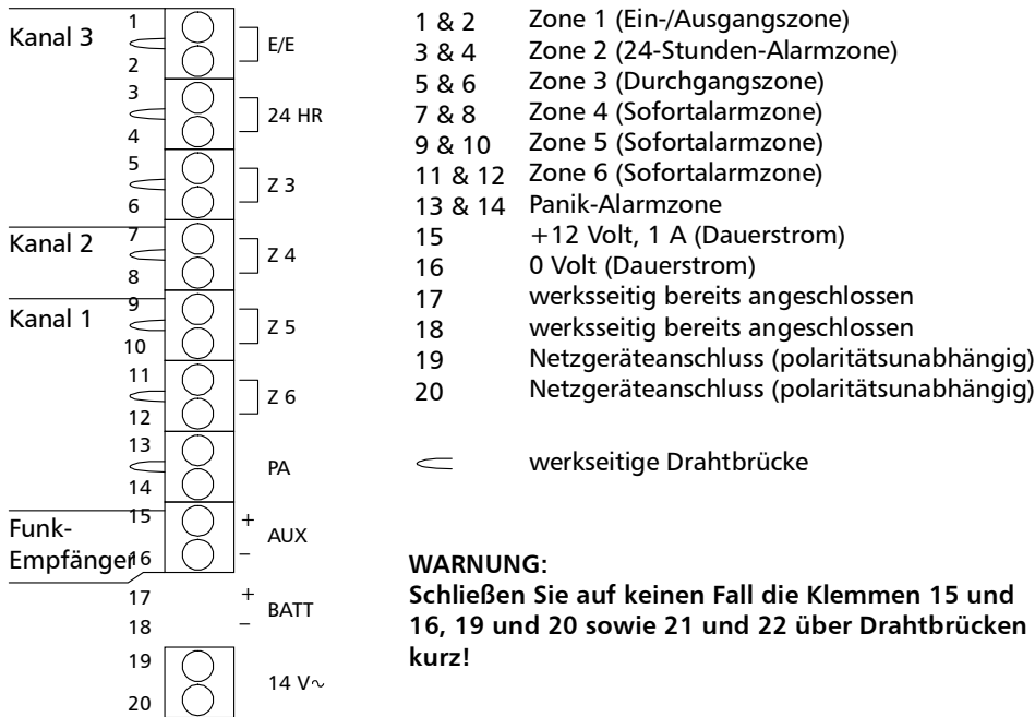
Abb. 29 : Klemmenbelegung der Zentrale (inklusive der werkseitigen Drahtbrücken)
