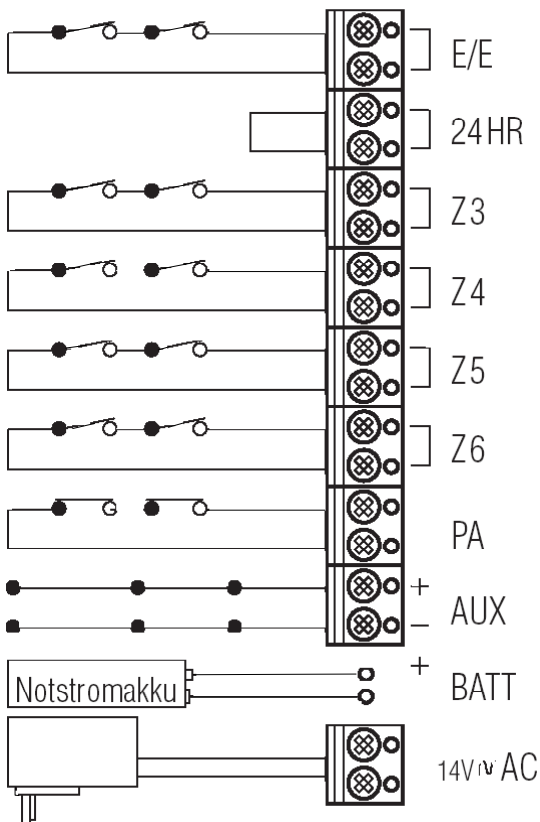
Abb. 30 : Anschluss Alarmzone (schematisch)
