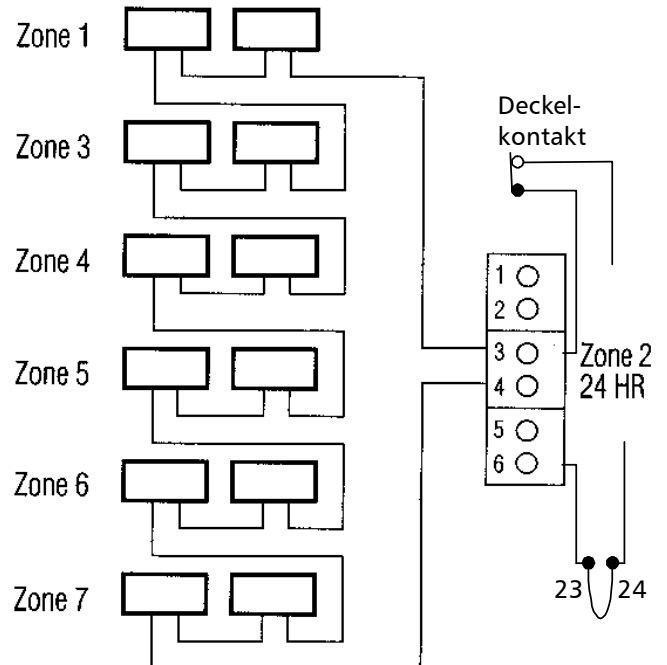
Abb. 31 : Anschluss Sabotagekreis (schematisch)
