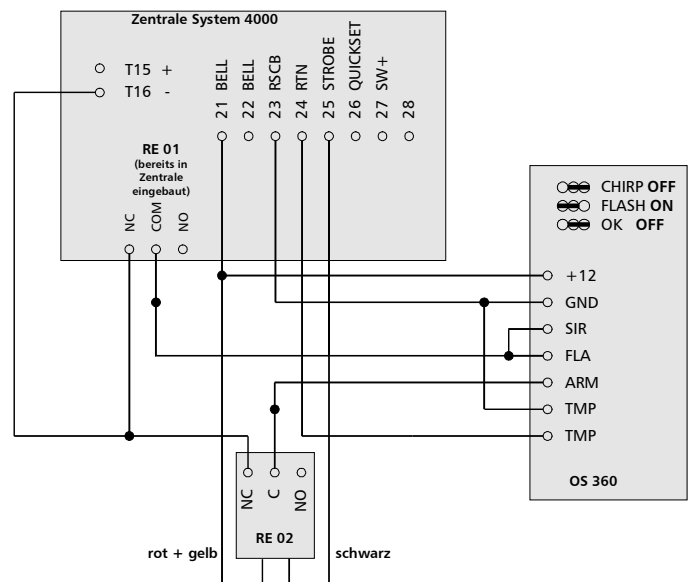
Abb. 25 : Beispiel mit OS 360 Relaismodul RE 02 in der Zentrale anschließen
