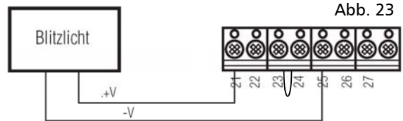
Anschluss eines Blitzlichtes
